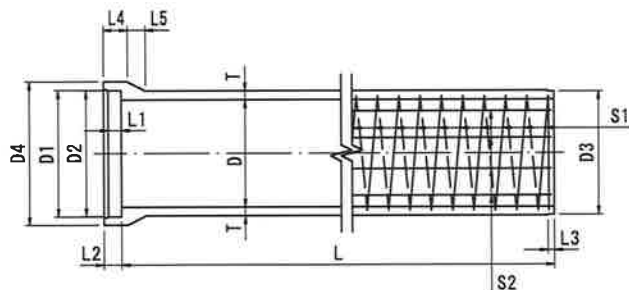
B形管
