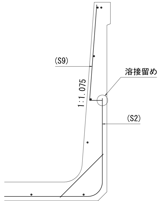
断面図
