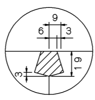
目地詳細図
