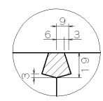
目地詳細図
