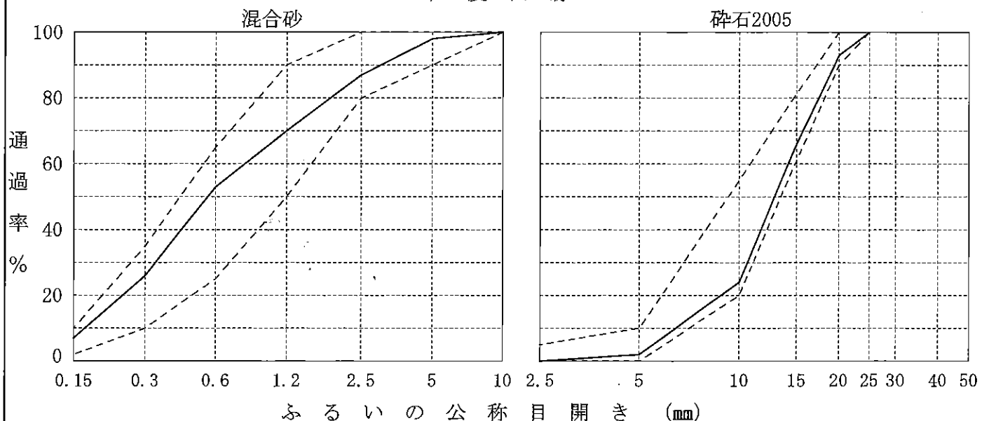
粒度曲線
