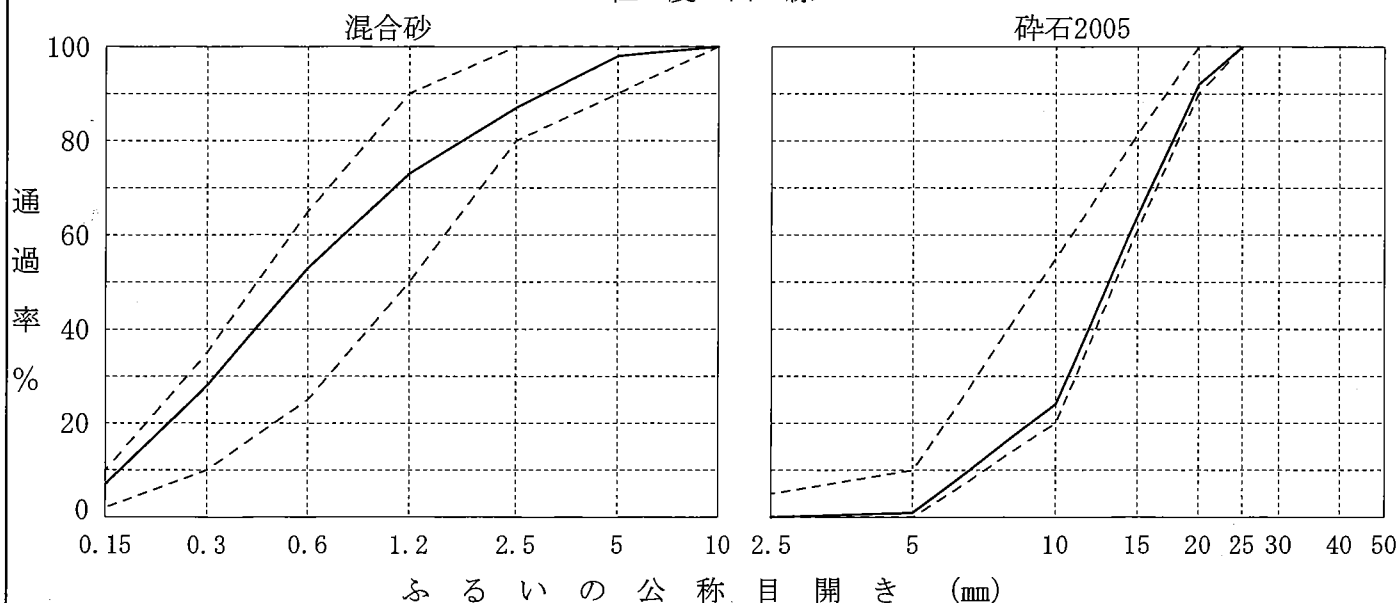
粒度曲線
