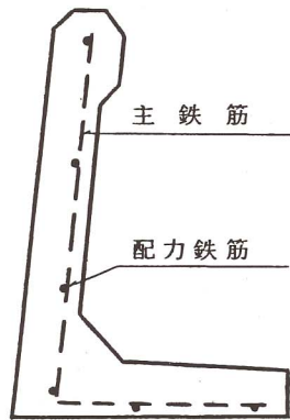
配筋図
