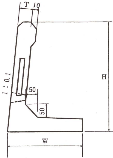
配筋図
