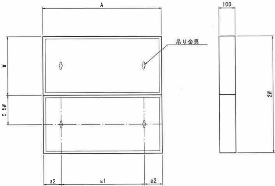
吊り金具詳細図 S=1:1
