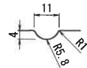
凹模様部詳細図
