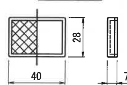
反射板詳細図
