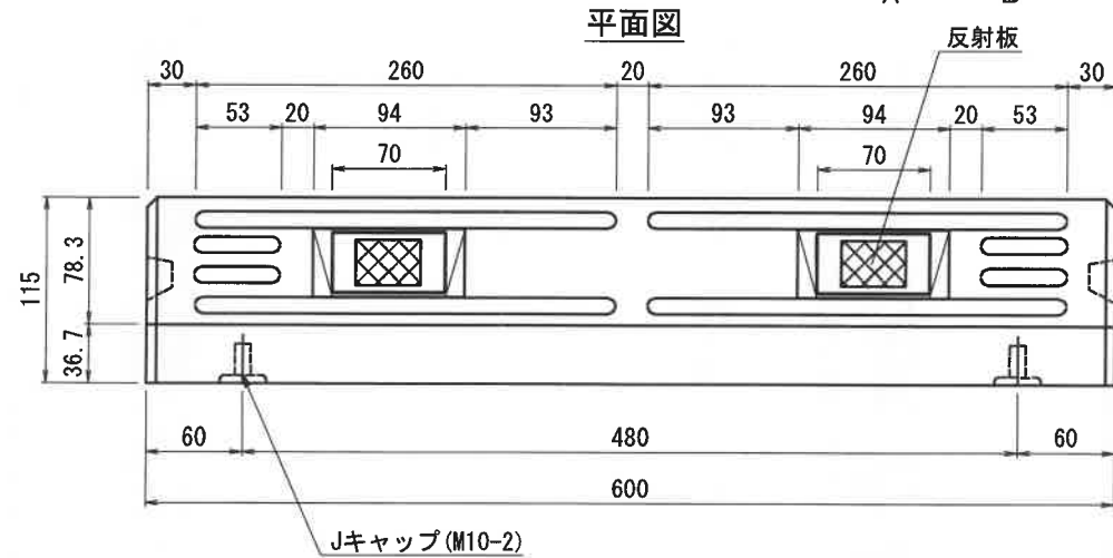
反射板取付プレート詳細図
