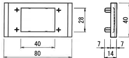
反射板取付プレート詳細図
