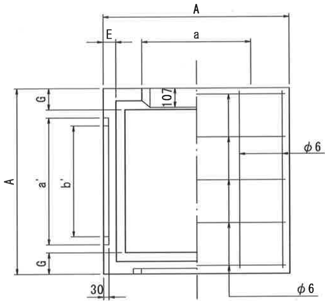
平面図
