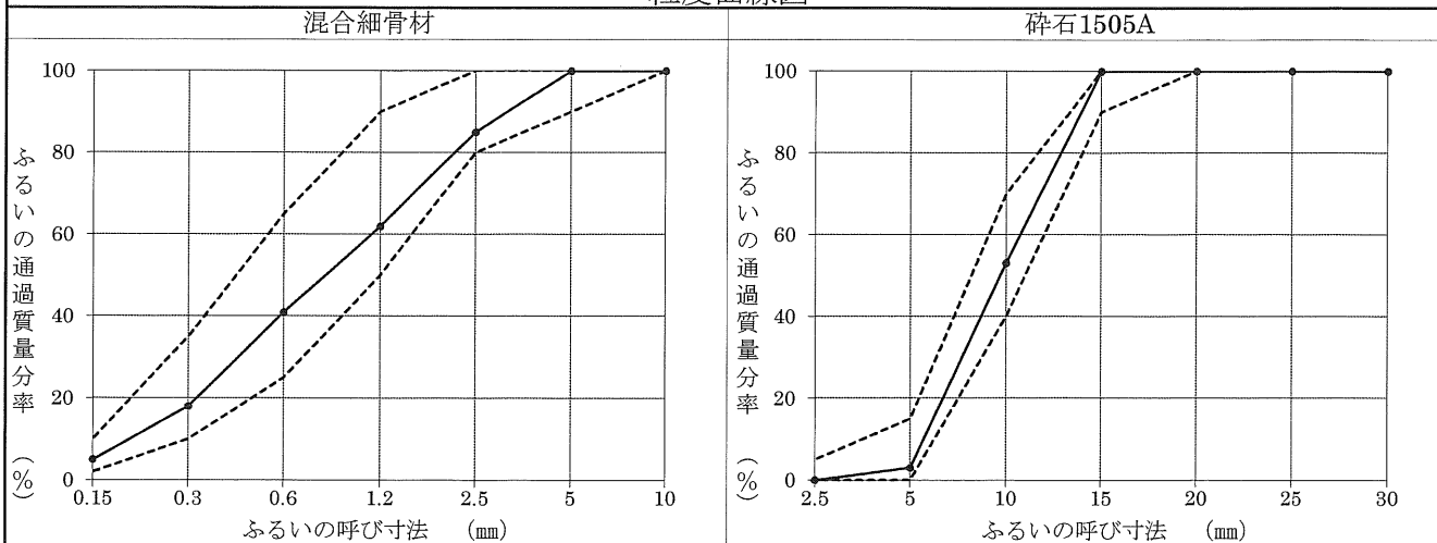
粒度曲線図
