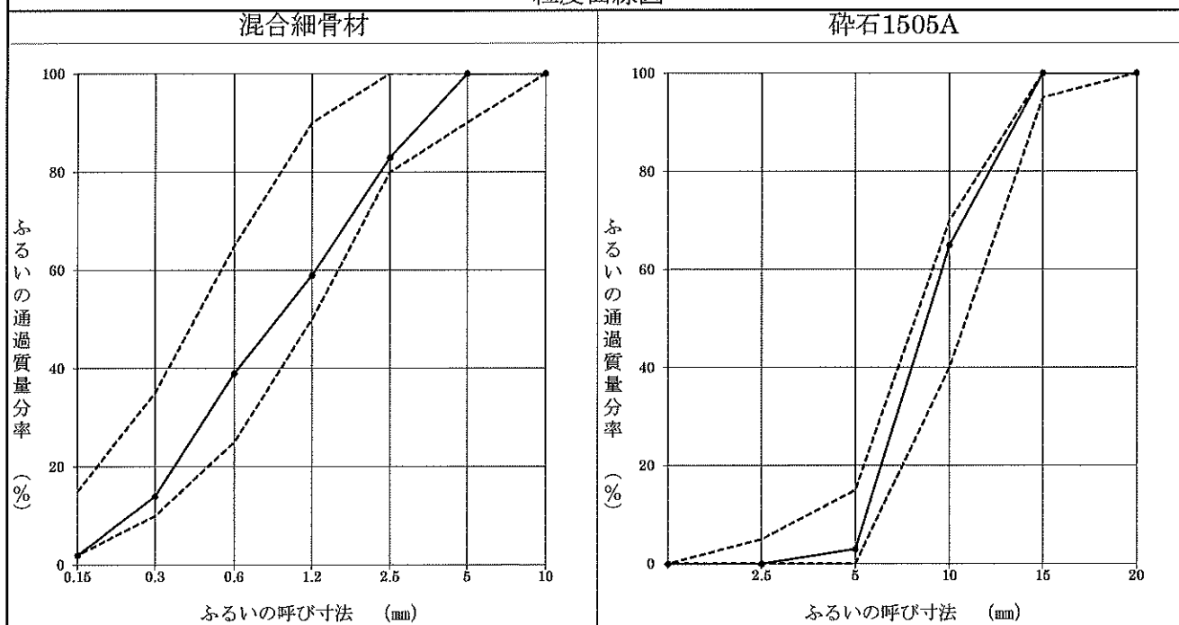
粒度曲線図
