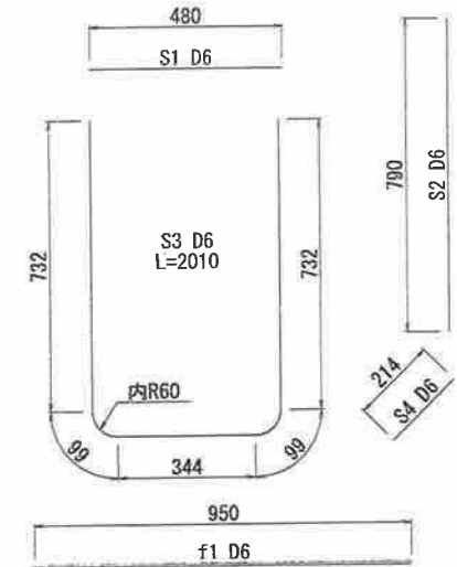
鉄筋加工図
