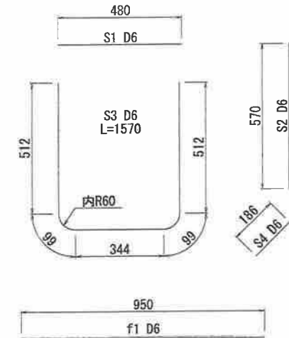
鉄筋加工図
