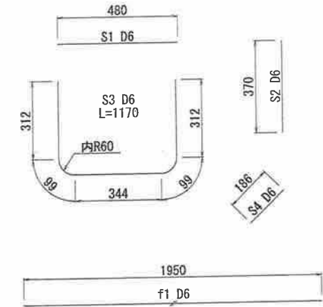
鉄筋加工図
