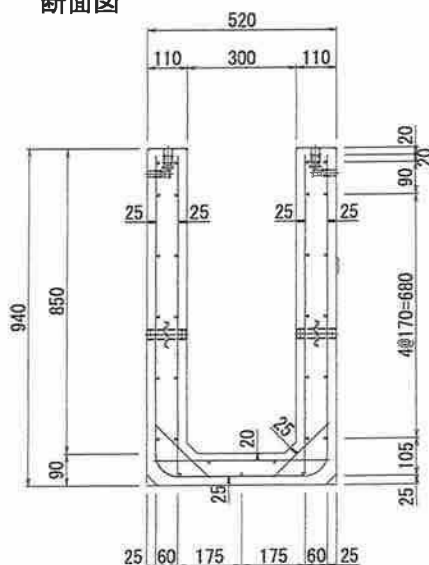
断面図
