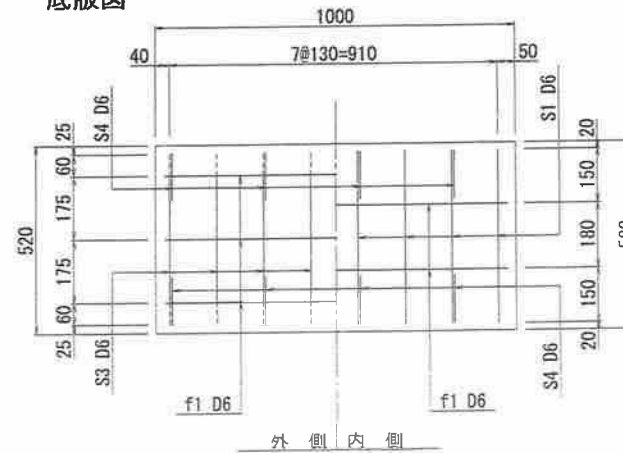
底版图
