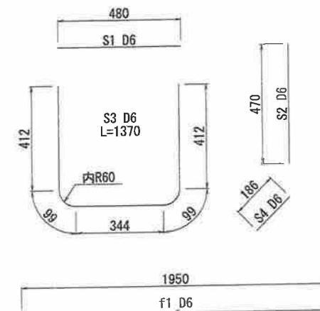
鉄筋加工図
