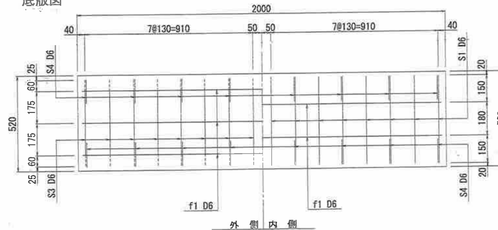
底版図
