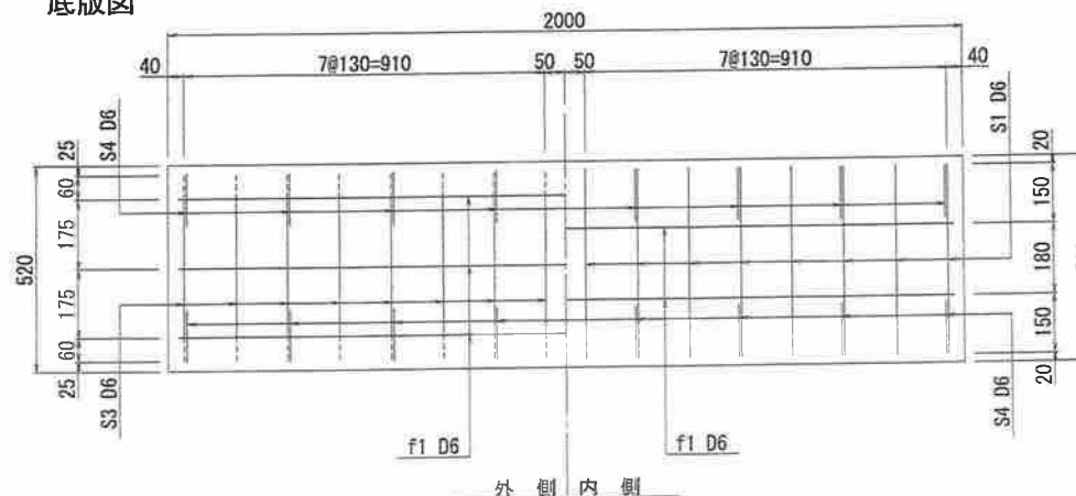
底板図
