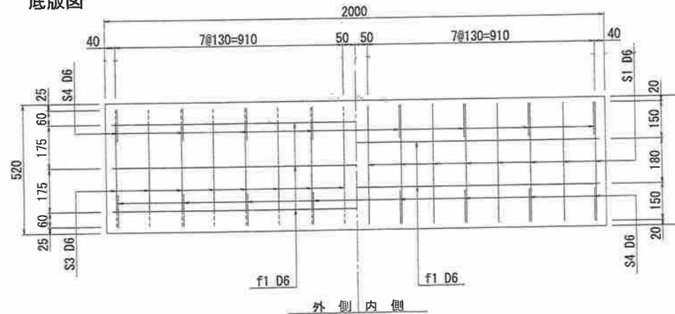
底版図
