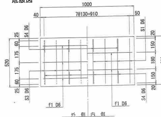
底板図
