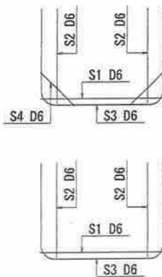
鉄筋組立図
