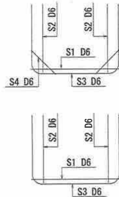
鉄筋組立図
