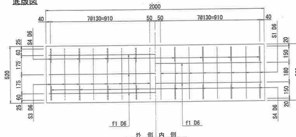
底板図
