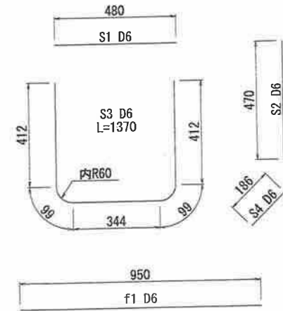
鉄筋加工図
