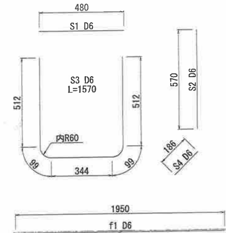
鉄筋加工図
