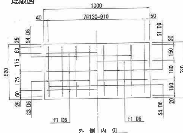
底版図
