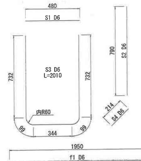
鉄筋加工図
