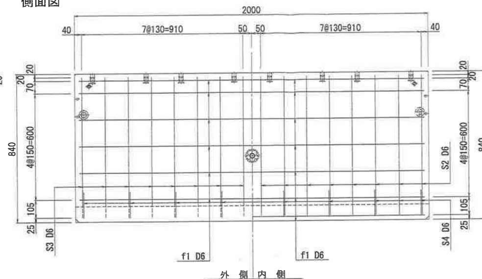
底板図
