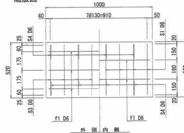
底版図
