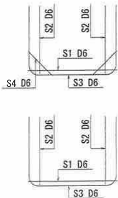
鉄筋組立図
