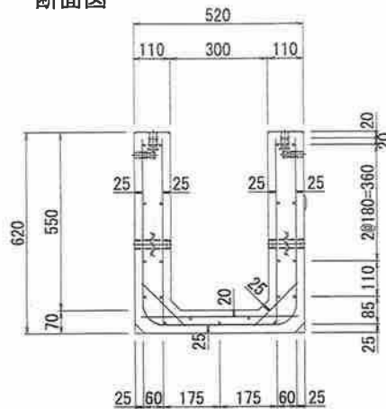
断面図
