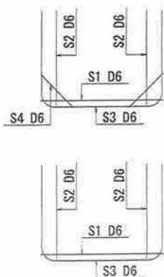
鉄筋組立図
