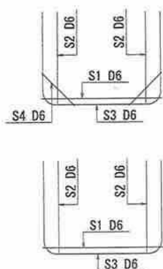
鉄筋組立図
