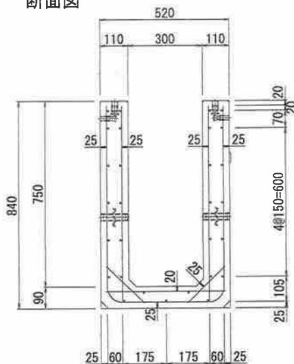
断面図
