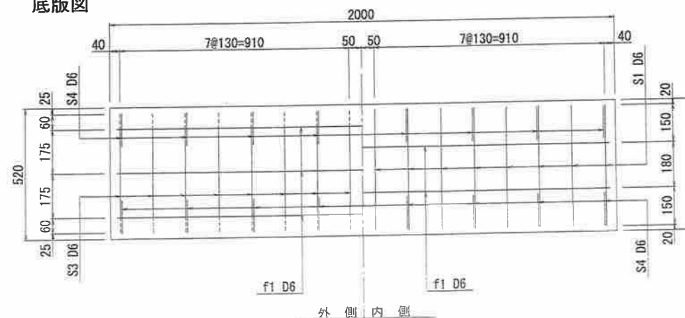
底版図
