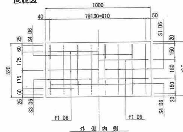
底板図
