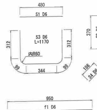
鉄筋加工図
