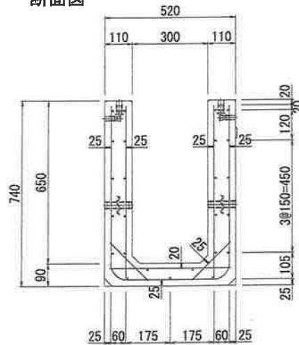
断面図
