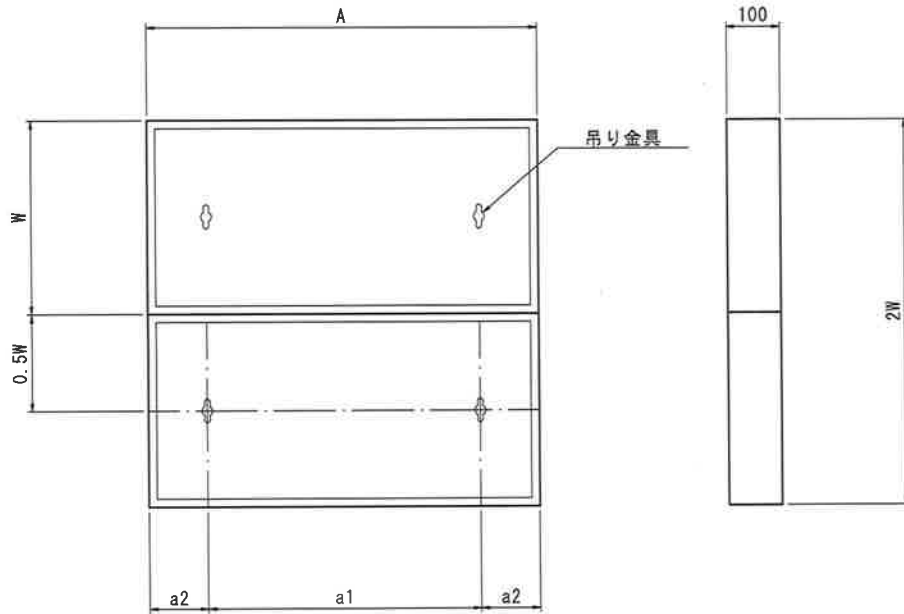
吊り金具詳細図
