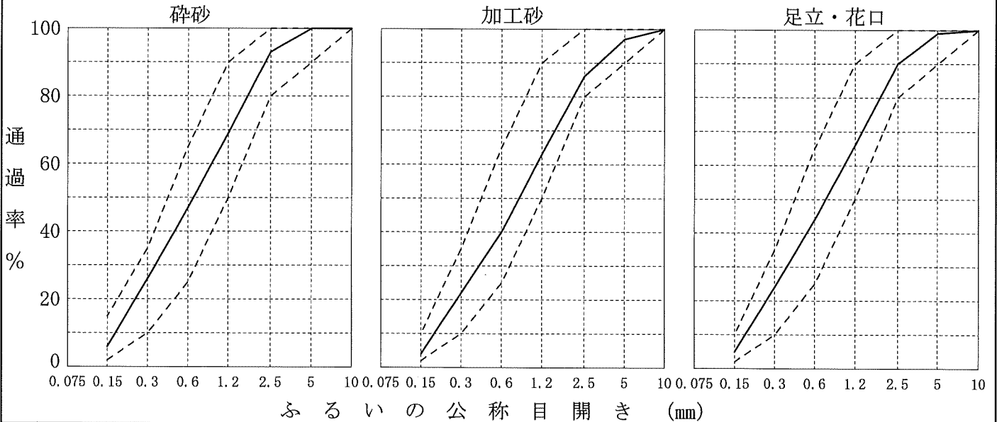
粒 度 曲 線
