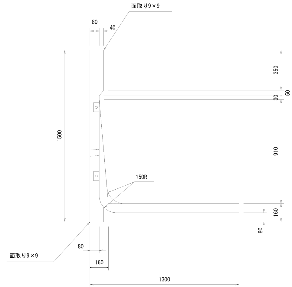
A-A断面図
