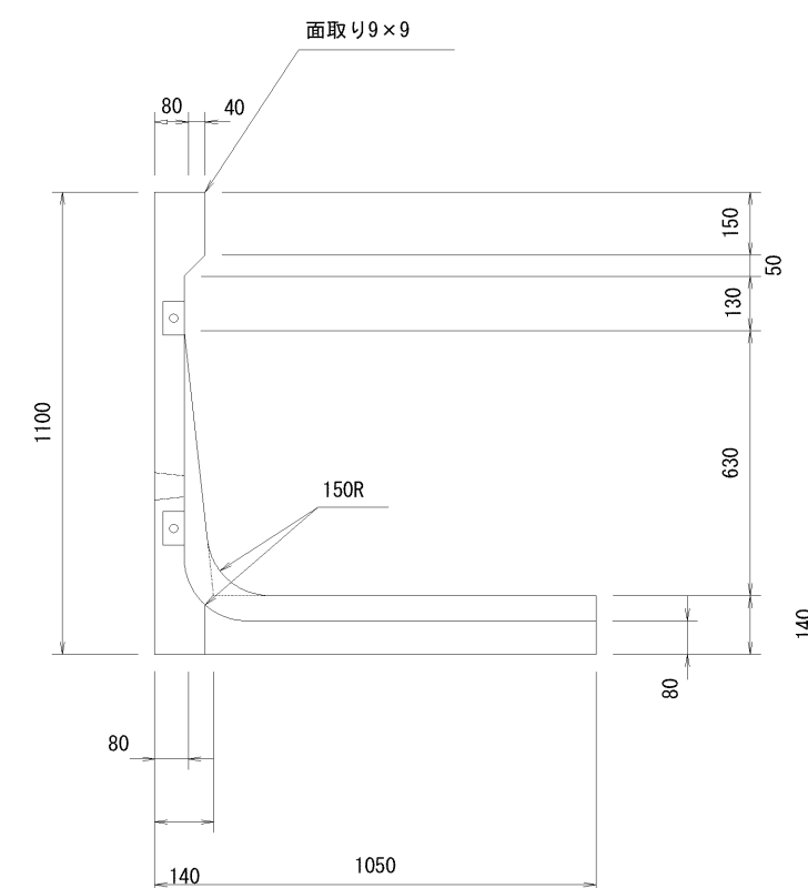
A-A断面図
