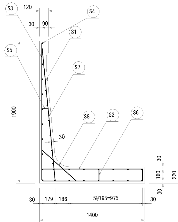
材料表
