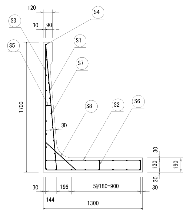
材料表
