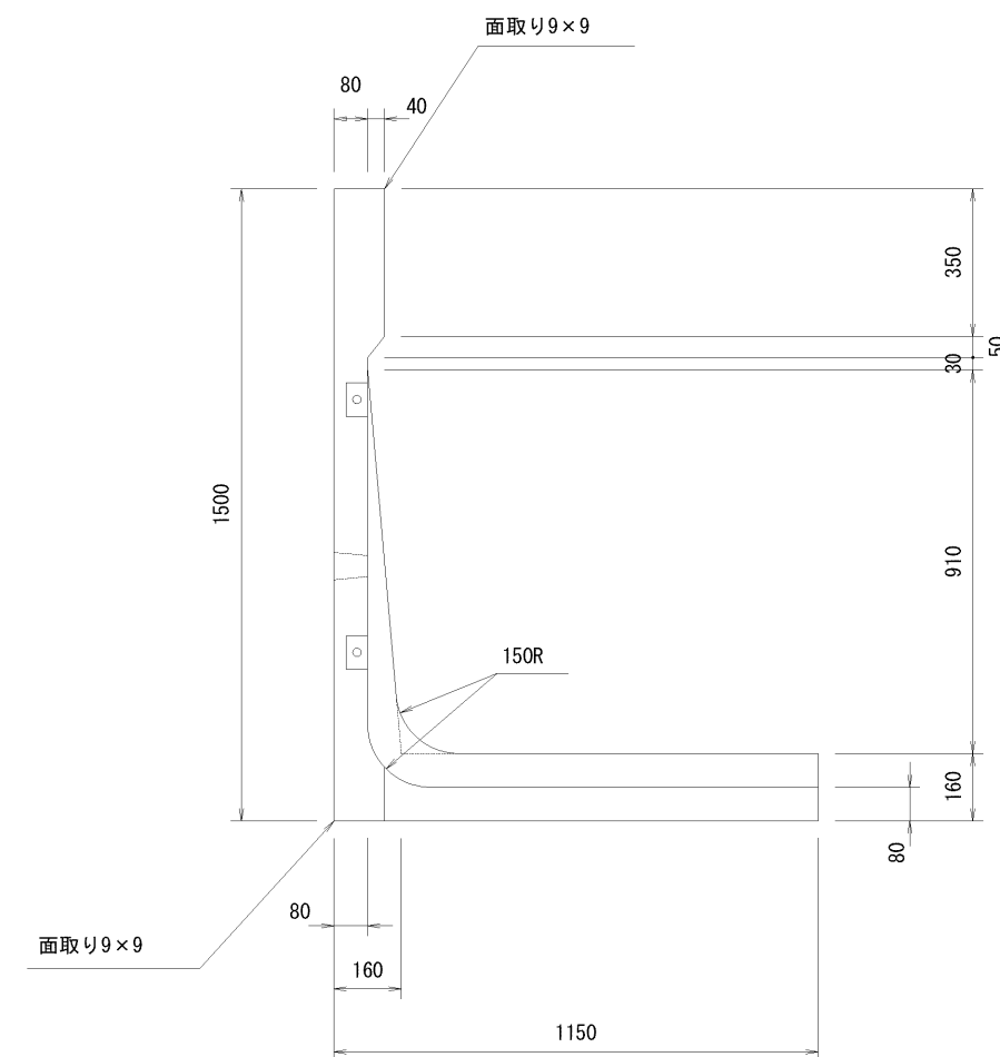
A-A断面図
