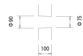
A-A断面図
