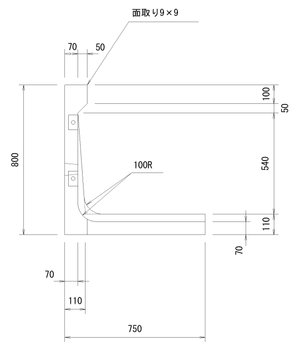
A-A断面図
