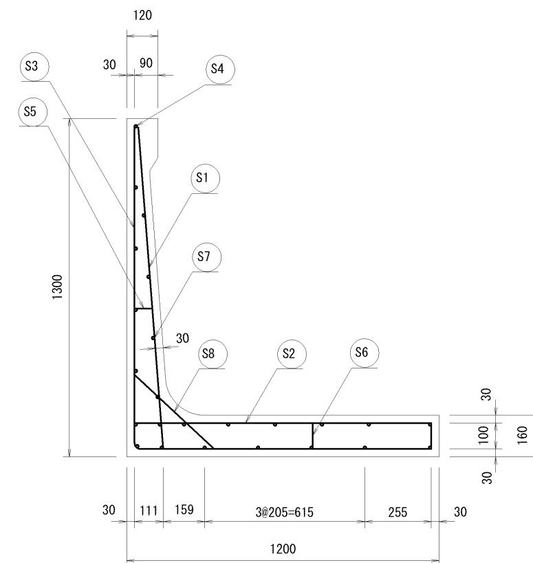
材料表
