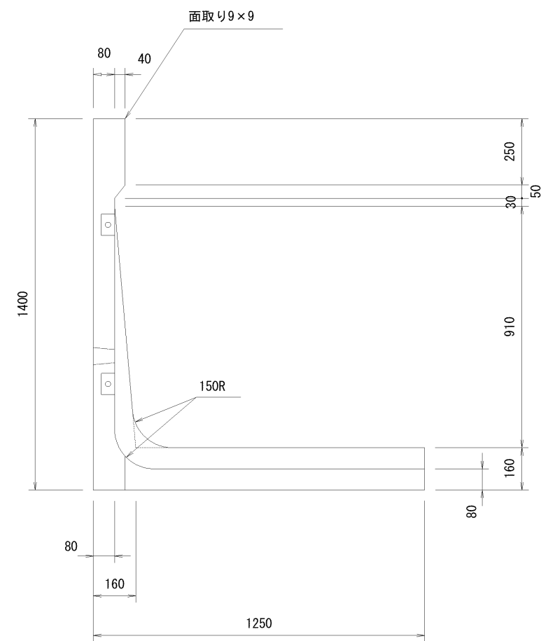
A-A断面図
