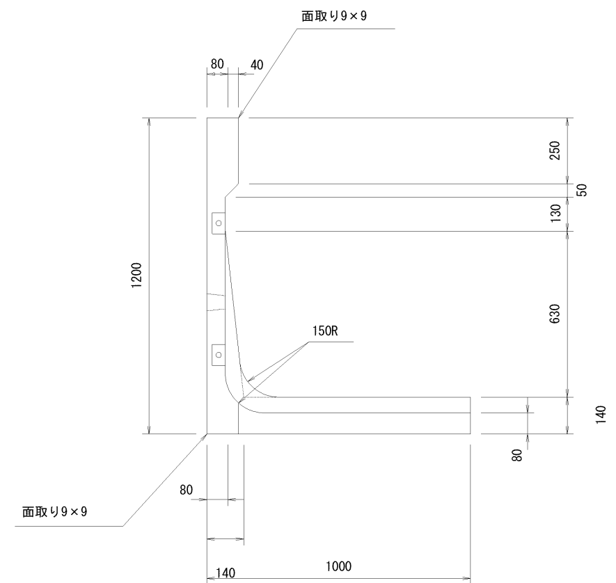
A-A断面図
