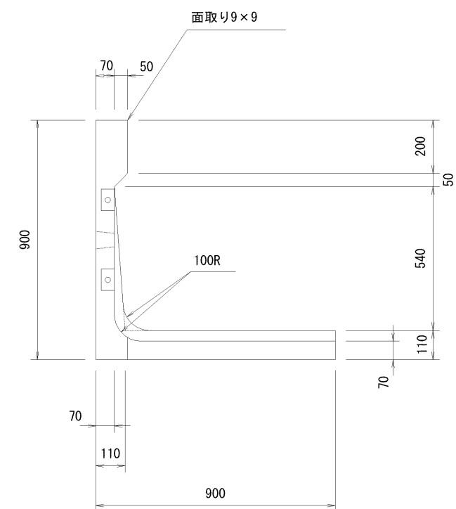
A-A断面図
