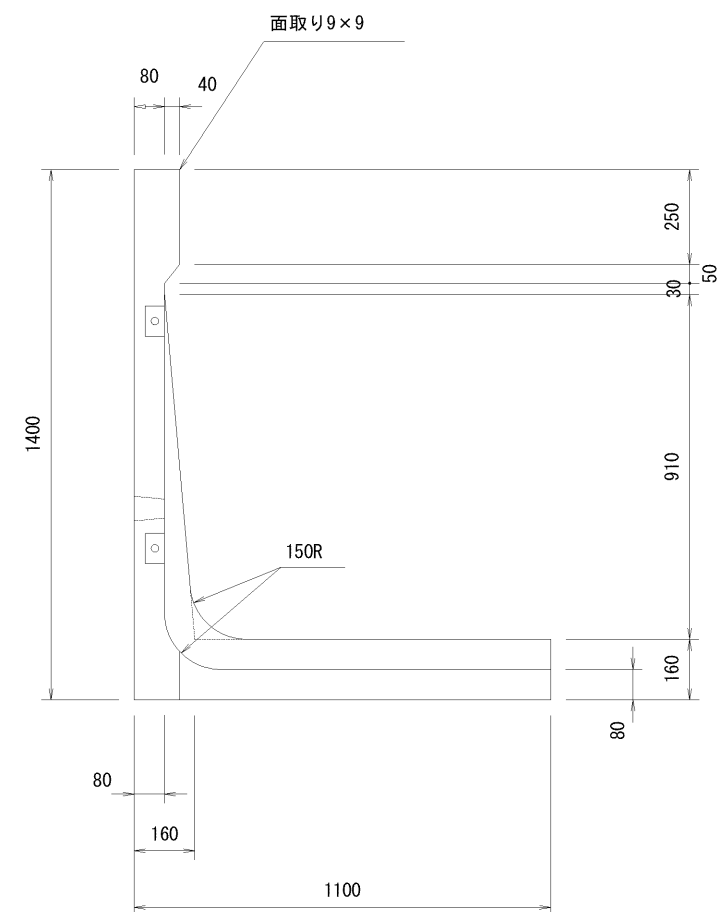
A-A断面図
