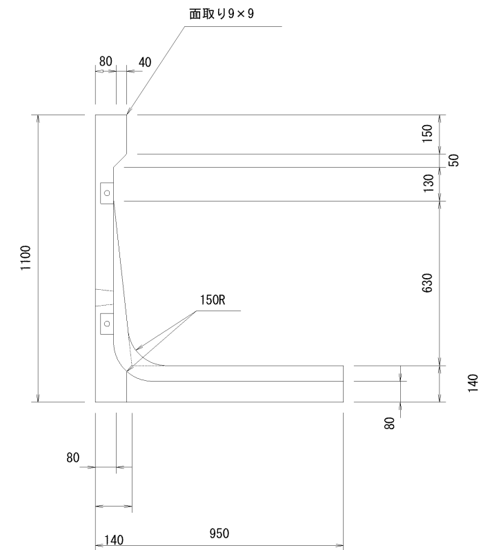
A-A断面图
