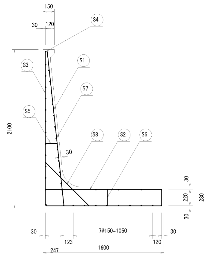
材料表
