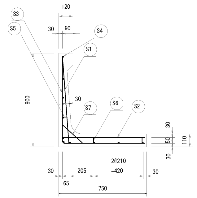
材料表
