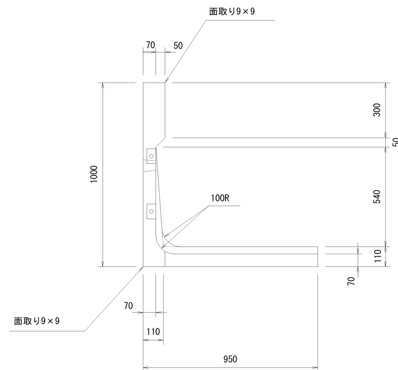
A-A断面図
