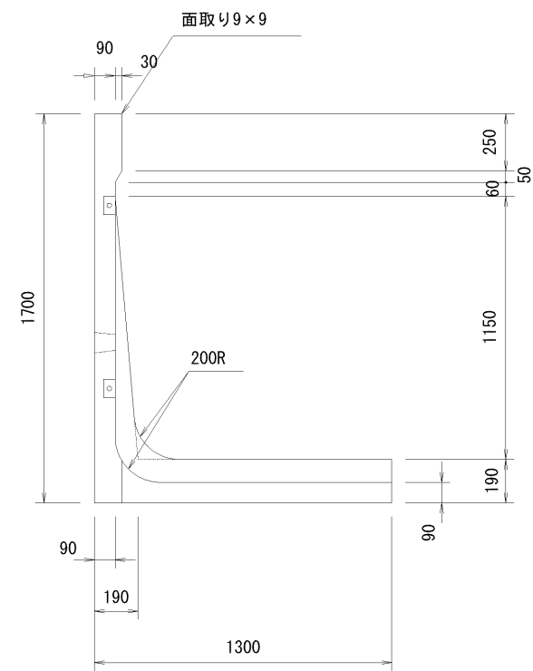
A-A断面図
