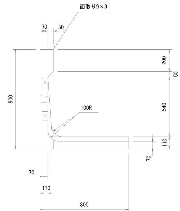
A-A断面図
