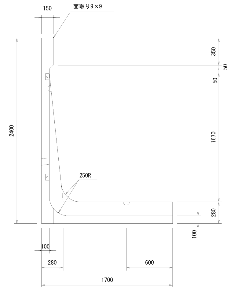
A-A断面図
