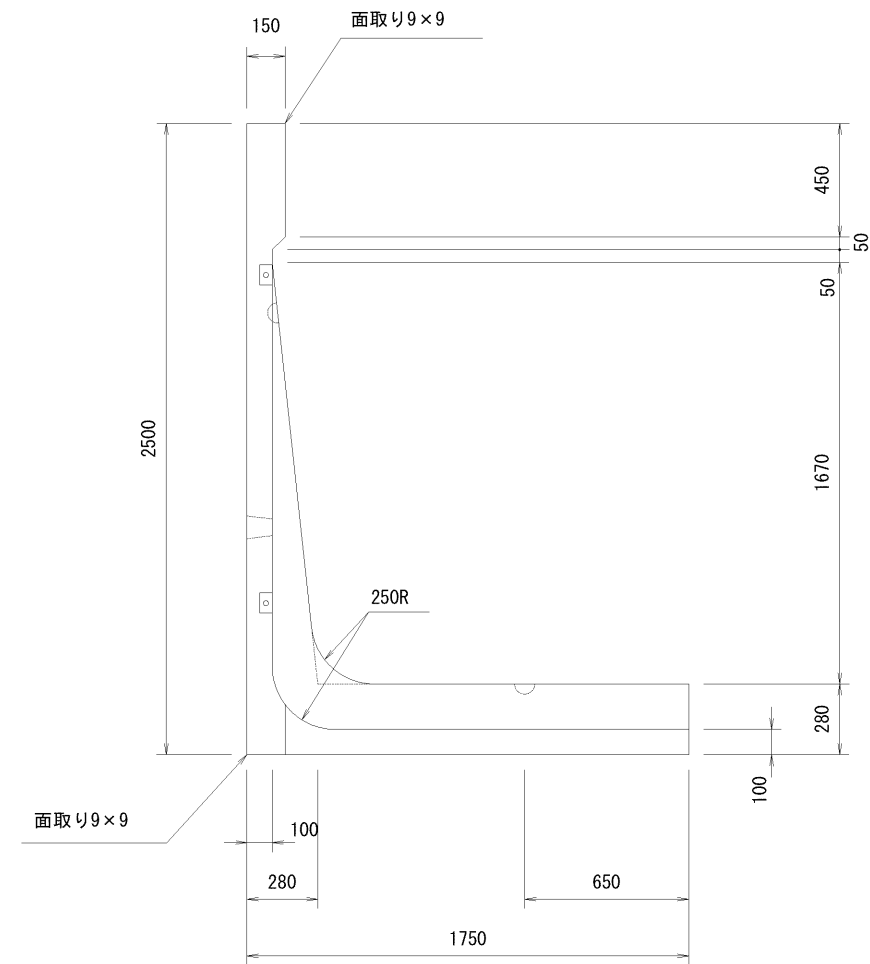
A-A断面図
