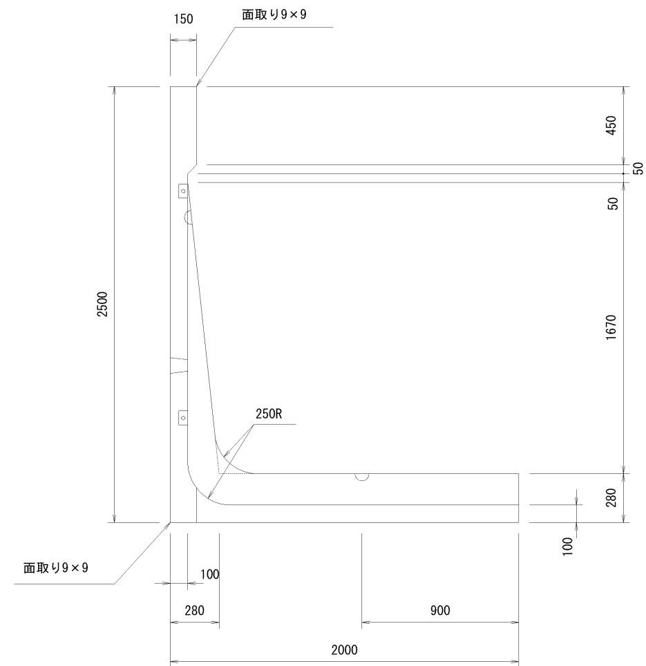
A-A断面図
