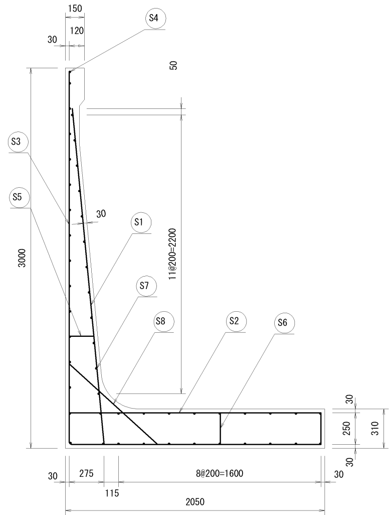
材料表
