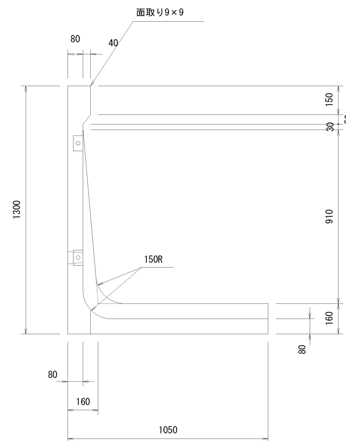
A-A断面図
