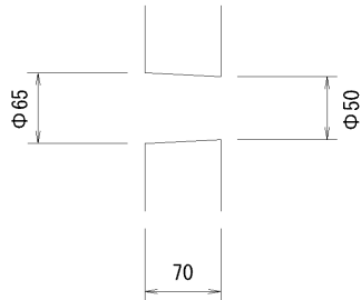
A-A断面図
