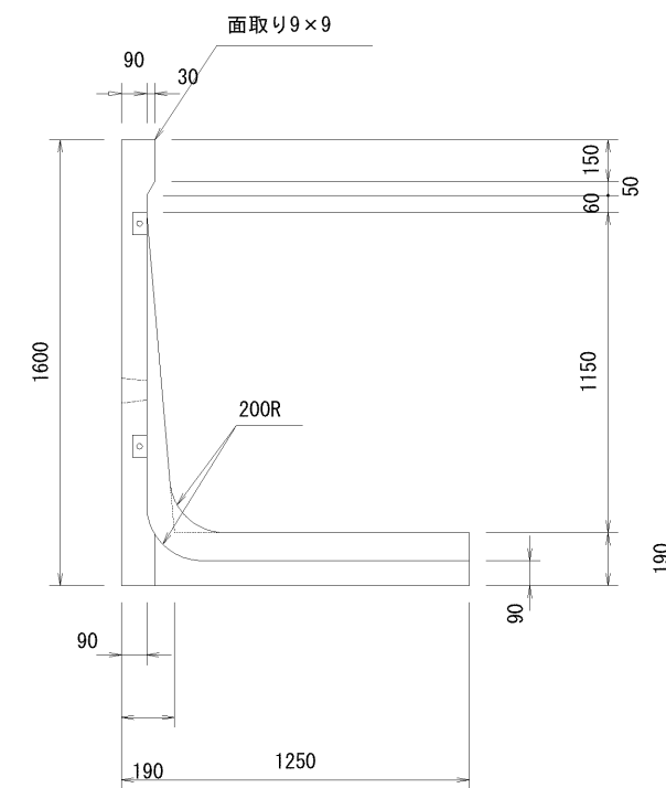
A-A断面図
