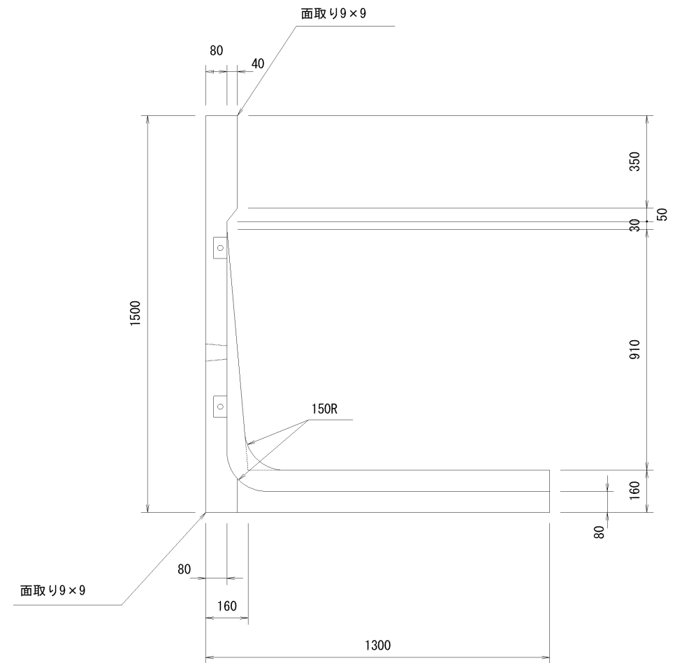
A-A断面図
