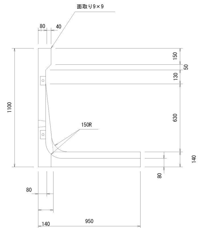
A-A断面図
