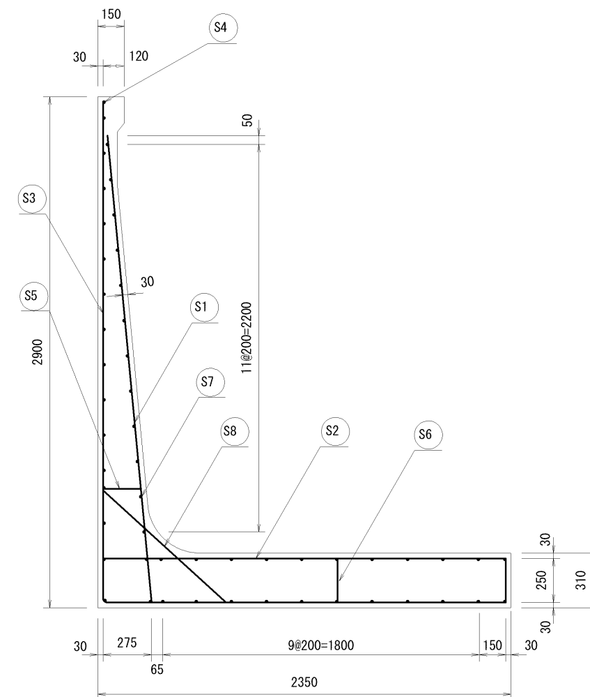
材料表
