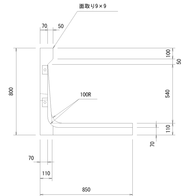
A-A断面図
