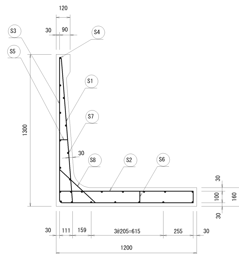
材料表
