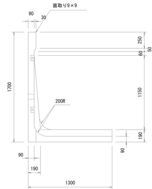
A-A断面図
