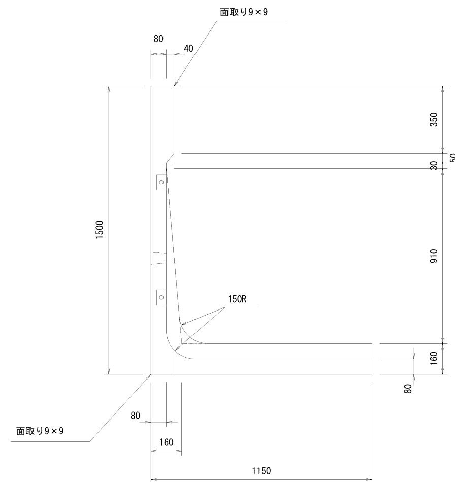
A-A断面図
