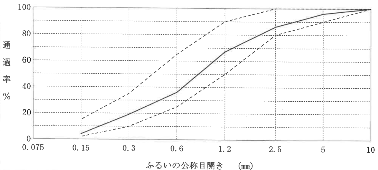
粒度曲線
