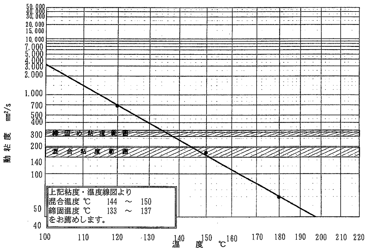
温度 - 粘度 図
