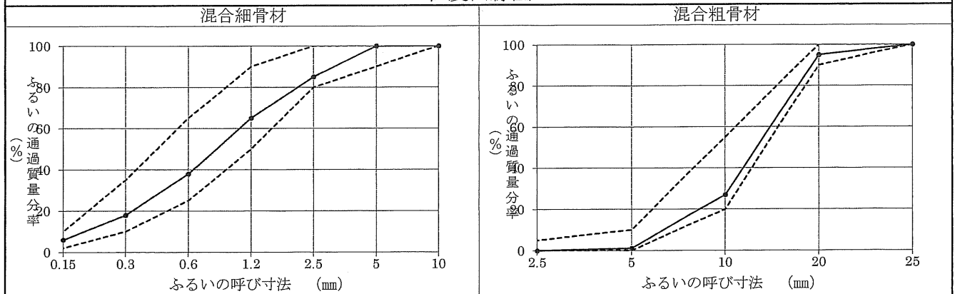
粒度曲線図
