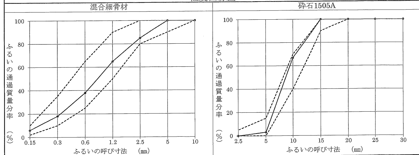
粒度曲線図
