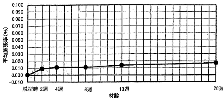
図-1 平均膨張率と材齢の関係
