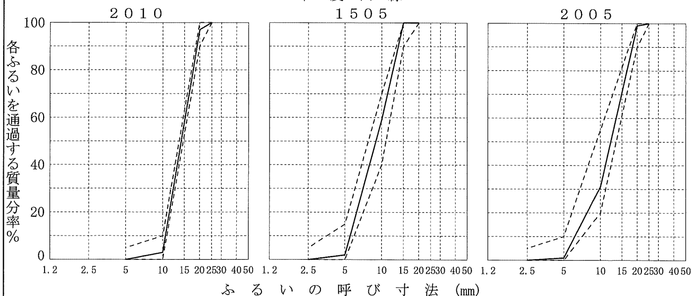
粒 度 曲 線
