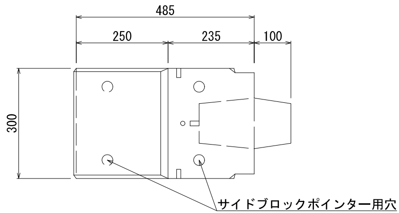
側面図
