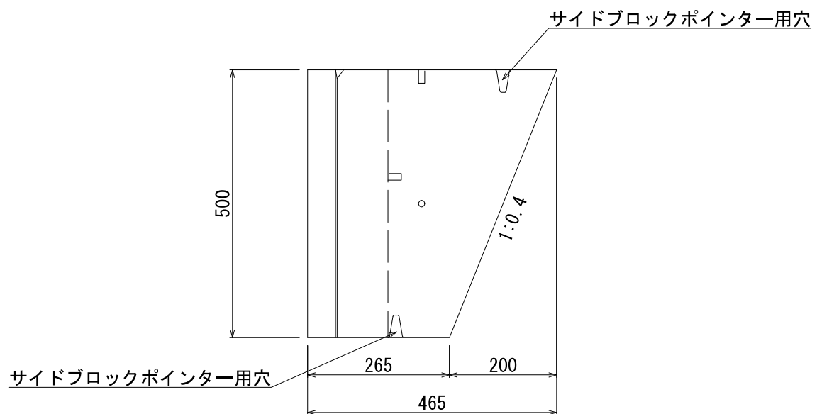
側面図
